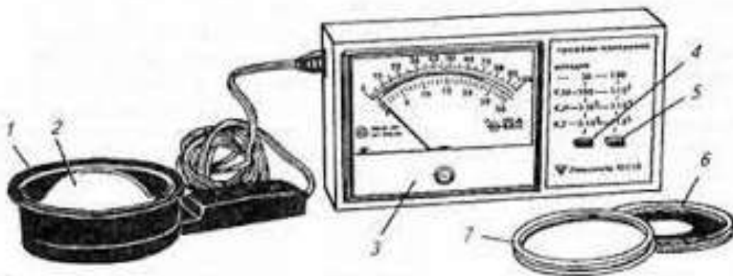
Рис.1 Люксметр Ю-116: 1 - корпус фотоелементу, 2 - насадка К; 3 - вимірювач; 4,5 - відповідно кнопки нижньої і верхньої шкали вимірювача; 6, 7 - насадки М, Р або Т
