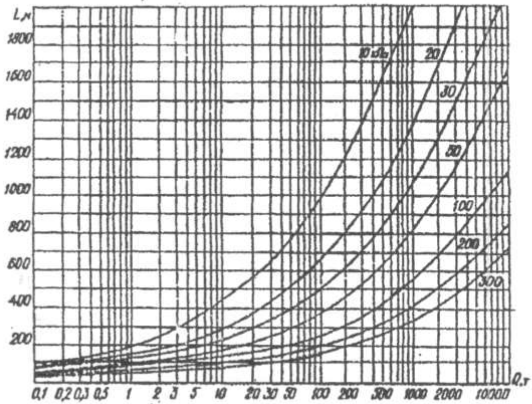
Рис. 1. Графіки надмірного тиску в залежності від маси пропану і відстані до центру вибуху
